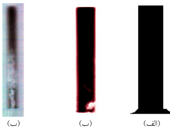
شکل ۵- تصاویر رادیوگرافی از نمونه‌های حاوی: (الف) حاوی ۱۵ درصد حجمی TiC در قالب سرامیکی، وضعیت نمونه سالم (ب) ۱۵ درصد حجمی TiC در قالب مسی، وضعیت نمونه: دارای تخلخل (پ) ۵ درصد حجمی TiC در قالب مسی، وضعیت نمونه: سالم
