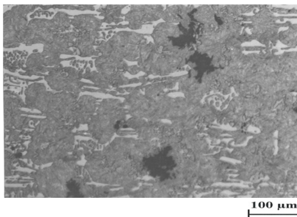
شکل ۶- تشکیل گرافیت برفکی شکل در نمونه آنیل شده Fe-10% Ti-3% C: ساختار زمینه پرلیت، شرایط عملیات حرارتی: گرم کردن نمونه تا 950^{\circ}\text{C} به مدت ۱ ساعت و سرمایش در هوا، ابعاد نمونه: نمونه‌های استوانه‌ای به قطر ۱/۵ و طول ۵ سانتی متر
