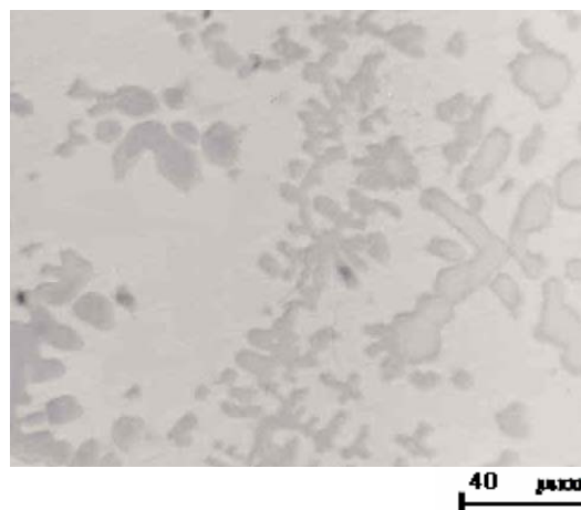
شکل ۳- خوشه‌ای شدن ذرات کاربیدی در نمونه Fe-10%Ti-3 %C ریخته‌گری شده به روش گریز از مرکز در قالب سرامیکی پیش‌گرم شده در دمای ۴۰۰ درجه سانتیگراد، در حالت اچ نشده
