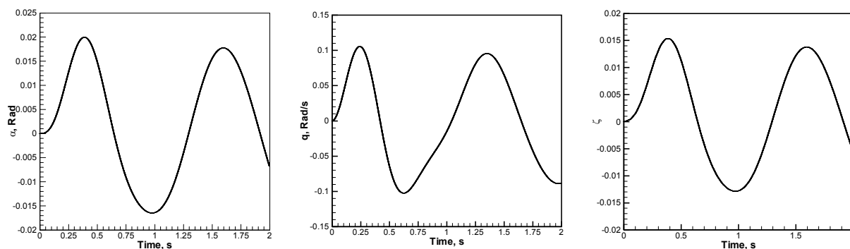
شکل ۷- پاسخ سیستم به ورودی پله برای سطح کنترلی در سرعت ۱۰۰۰ m/s با فرکانس پنج هرتز
