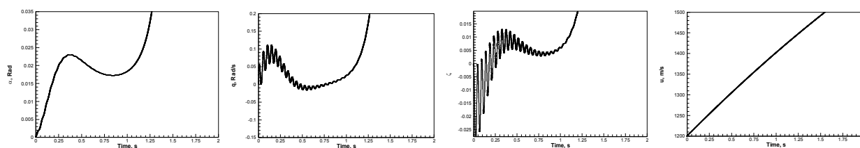
شکل ۱۰- پاسخ سیستم به تندباد با وجود نیروی پیشروان ۳۰ kN
