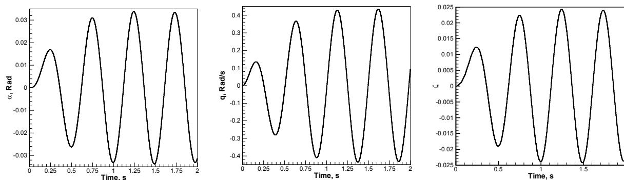
شکل ۸- پاسخ سیستم به ورودی نوسانی برای سطح کنترلی در سرعت ۱۰۰۰ m/s با فرکانس سیزده هرتز
