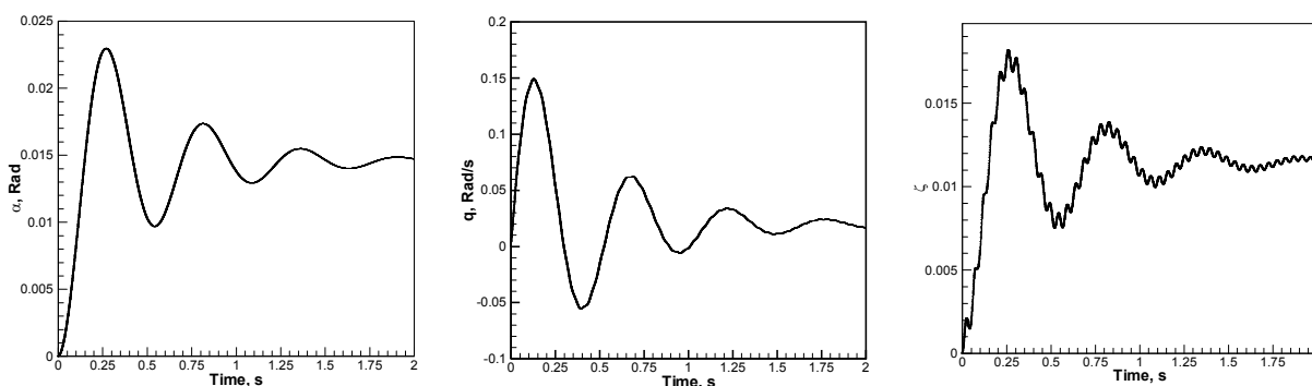
شکل ۶- پاسخ سیستم به ورودی پله برای سطح کنترلی در سرعت ۱۰۰۰ m/s
