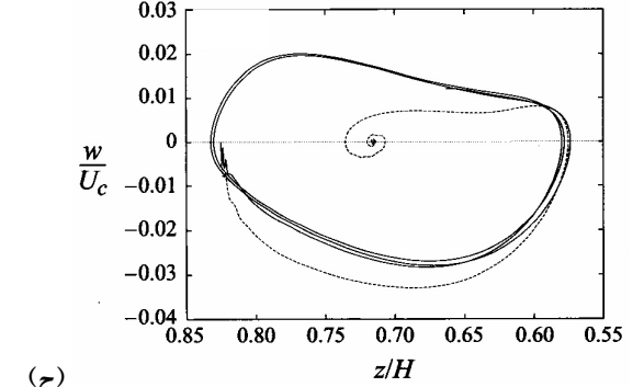
شکل ۱۱- مولفه سرعت w نسبت به مختصات z یک قطره در چهار عدد رینولدز متفاوت: الف) Re=10 ، ب) ۲۵، ج) ۳۷ و د) ۵۰. پارامترهای دیگر جریان عبارت اند از: We=0/5 ، \alpha=8
