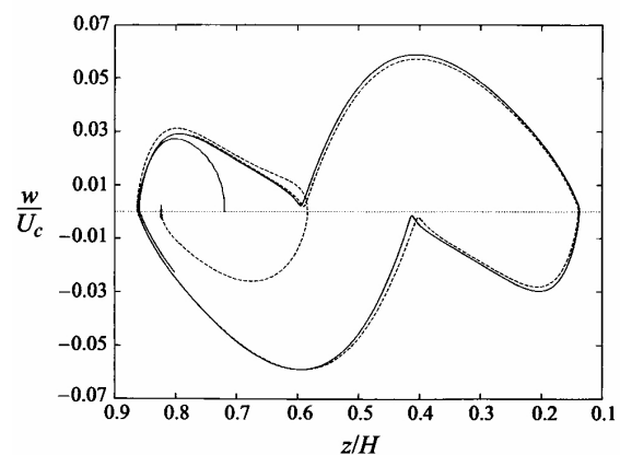
شکل ۱۲- مولفه سرعت w بر حسب مختصات z دو قطره با موقعیت اولیه متفاوت در \gamma=1 ، \alpha=8 ، Re=37 و We=0.5 . خطوط پر مربوط به یک قطره در یک موقعیت عرضی مشخص و خط چین مربوط به یک قطره با موقعیت عرضی متفاوت است
