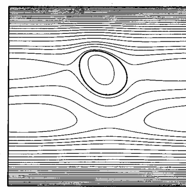
شکل ۷- خطوط جریان برای یک قطره در (\alpha=1, Re=1) ، (الف) (Ca=1, \gamma=1, We=1) و (ب) (Ca=2, \gamma=0.125, We=2)
