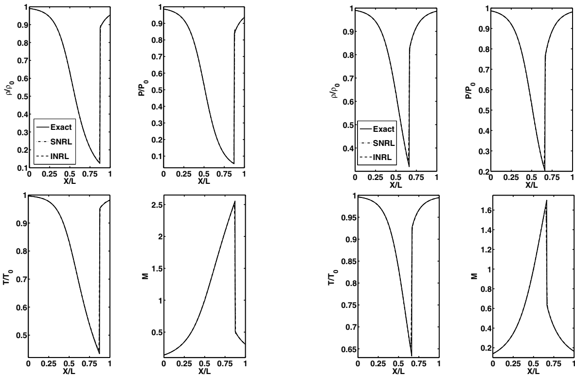
شکل ۷- مقایسه جوابهای تحلیلی با عددی به دست آمده از روش خطی سازی INRL و SNRL در کورانت ۰/۲ در شیپوره ۱ با فشار خروجی ۸۵ کیلو پاسکال
