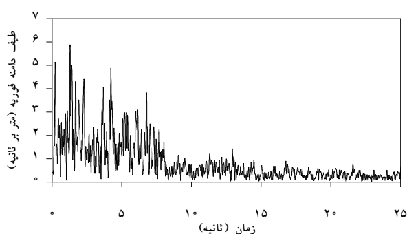
شکل ۵- طیف دامنه فوریه برای نگاشت "طبس"
