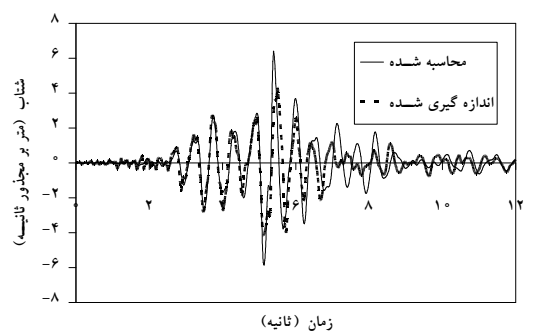
شکل ۲۰- تاریخچه شتاب افقی در اثر زلزله "ماموت لیک" در تاج سد "لانگولی"
