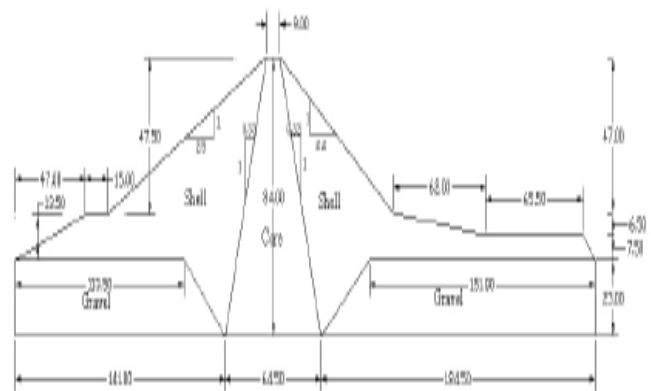
شکل ۱۰- مشخصات مقطع عرضی سد "سانتافله سیا" [۶]
