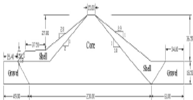
شکل ۱۴ - مشخصات مقطع عرضی سد "لانگولی"
