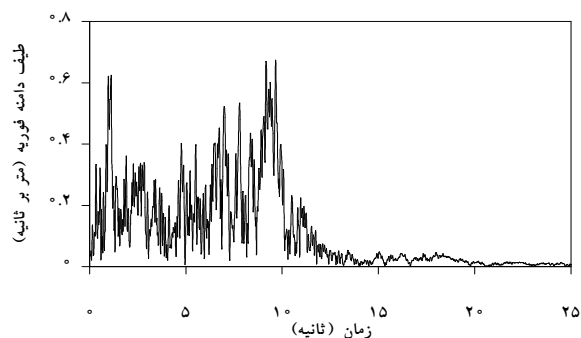
شکل ۷- طیف دامنه فوری برای نگاشت "سانفراندو"
