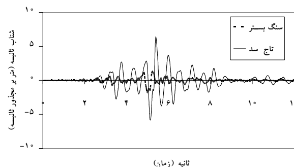
شکل ۲۲- تاریخچه شتاب افقی سنگ بستر و تاج سد "لانگولی"
