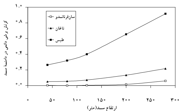
شکل ۳۴- رابطه بین کرنش برشی دائمی در دامنه سد نسبت به ارتفاع سد در اثر سه زلزله مشخص
