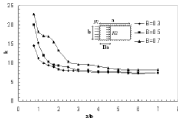
شکل ۶ - نمودار تغییرات ضریب کمانش موضعی k ( k = k_2 ) نسبت به a/b هنگامی که N_1 = 0
