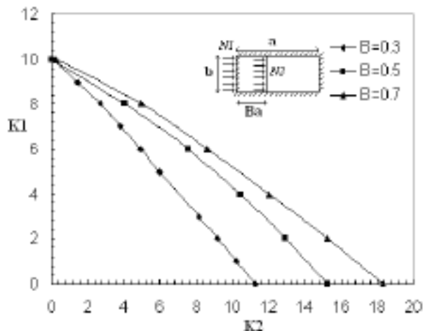
شکل ۸ - نمودار اندرکنش ضرایب کمایش k_1 و k_2 ( a=b )
