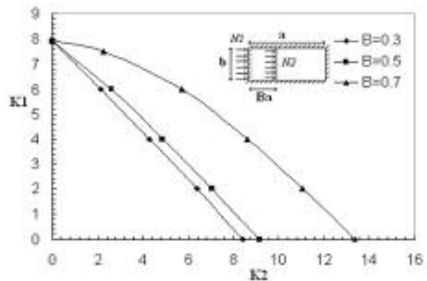
شکل ۱۰ - نمودار اندرکنش ضرایب کمایش k_1 و k_2 ( a=2b )
