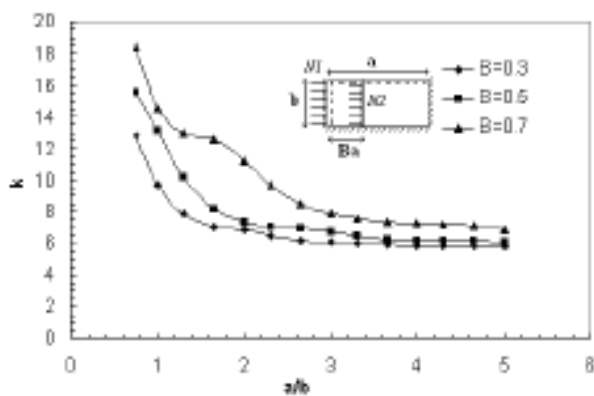
شکل ۹ - نمودار اندرکنش ضرایب کمایش
