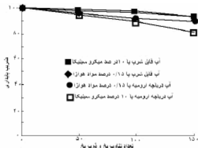
شکل ۱۴- مقایسه رفتار مخلوطهای مختلف در مقابل یخ و ذوب یخ در آبهای معمولی و دریاچه ارومیه
