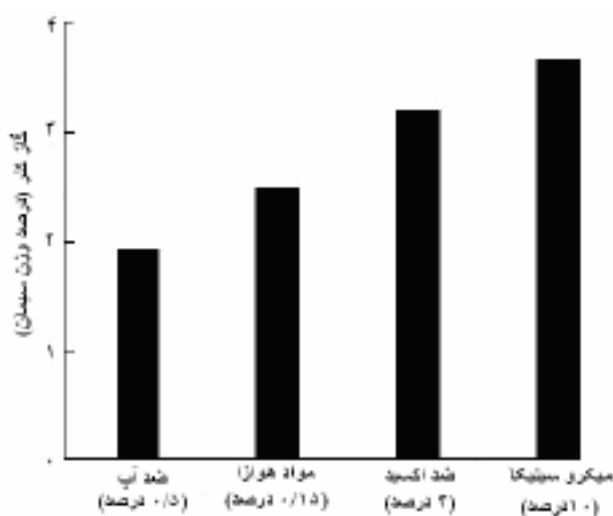
شکل ۹- تاثیر مقدار میکرو سیلیس و نوع سیمان بر مقدار نفوذ کلر
