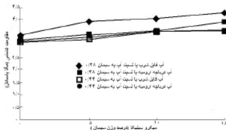
شکل ۳- مقاومت کششی ۲۸ روزه مخلوطهای دارای میکروسیلیس در آبهای معمولی و دریایچه ارومیه
