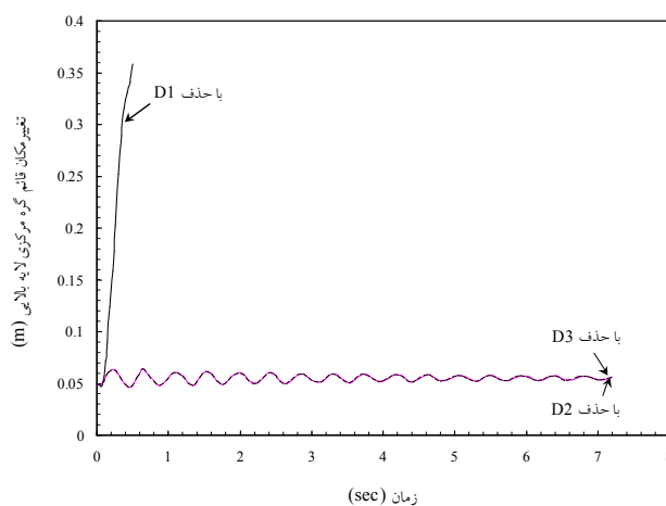
شکل ۱۲ - واکنش زمانی تغییر مکان گره مرکزی لایه بالایی سازه به ازای حذف هر یک از اعضای بحرانی جان
