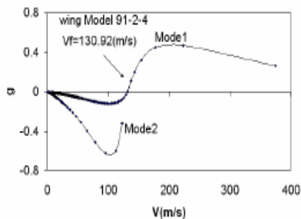
شکل ۵ - سرعت بر حسب g برای بال سری ۹۱-۴ آزمایش تجربی [۲۲] و روش حاضر
