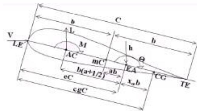
شکل ۱- نماد گذاری مقطع بال در راستای وتر
