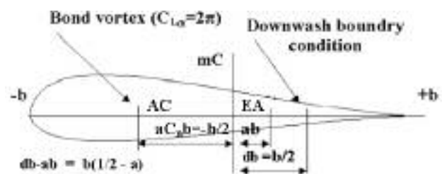
شکل ۳ - حالت تراکم ناپذیر با نماد مرجع [۳]
