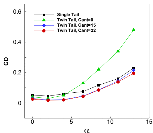
شکل ۵-ب) ضریب پسا
