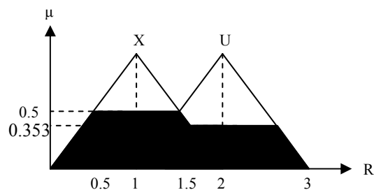
شکل ۸- خروجی فازی نرخ نزدیکی بین ماشینهای ۱ و ۲
