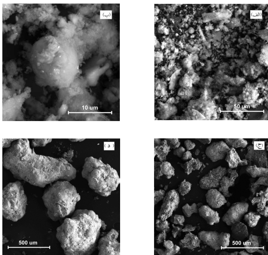
شکل ۹- تصاویر SEM ذرات پودر آلیاژ Al-۶wt%/Si (الف و ب) در گستره زیر ۳۸ میکرومتر، (ج) ۲۱۲-۱۰۶ میکرومتر و (د) ۵۰۰-۳۰۰ میکرومتر تهیه شده توسط سیکل (ب)
