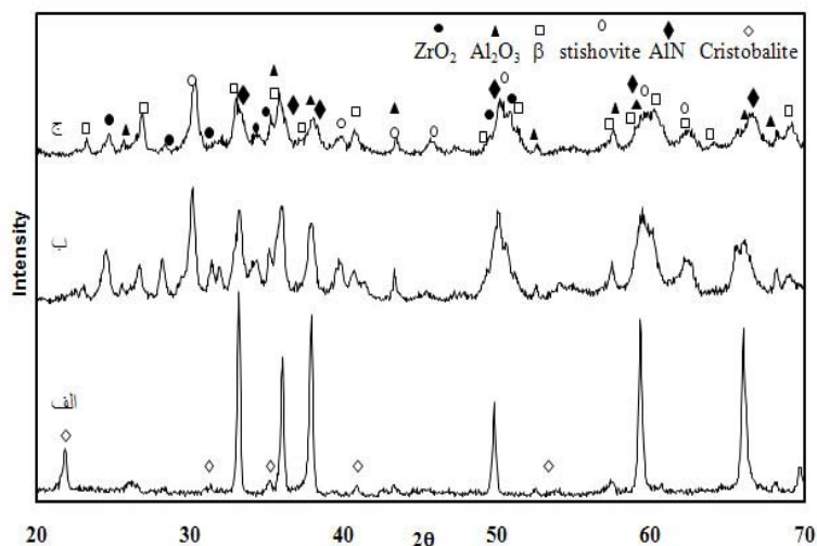
شکل ۹. الگوهای پراش پرتو ایکس از مخلوط پودر اکسید سیلیسیوم با نیتريد آلومينيوم پس از عمليات حرارتي در دمای 1200^{\circ}\text{C} به مدت ۲ ساعت، (الف) بدون آسیاب کاری، (ب) پس از ۱۰ ساعت آسیاب کاری و (ج) پس از ۲۰ ساعت آسیاب کاری.
