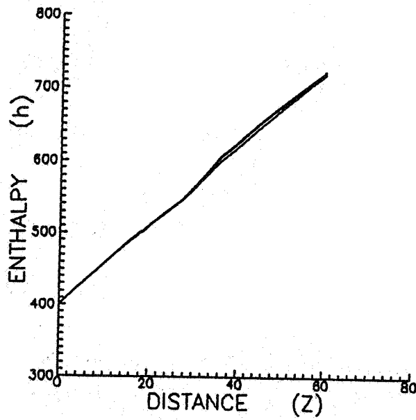
شکل ۷- تغییرات انتالی در طول کانال ۱
