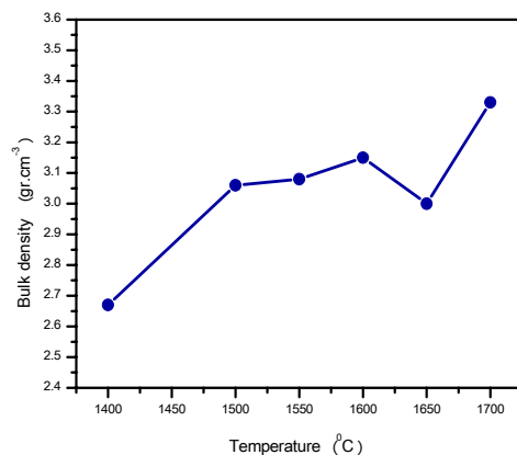
شکل ۷- تغییرات دانسیته کلی نمونه در دماهای مختلف زینتر
