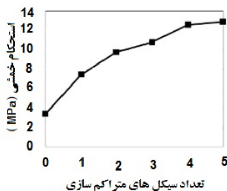
شکل ۶- تغییرات استحکام خمشی با افزایش تعداد سیکل‌های متراکم سازی کامپوزیت بر پایه چوب گردو
