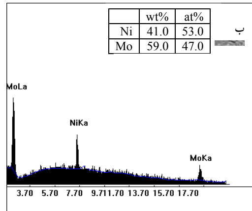
شکل ۶- (الف) تصویر SEM سطح شکست نمونه MN1.5، (ب) تحلیل EDS از نقطه مشخص شده در تصویر
