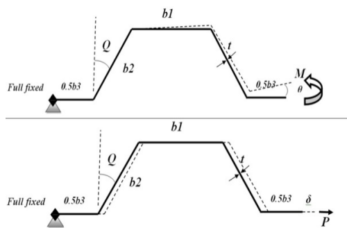
شکل ۲- پارامترهای المان دوزنقه ای
