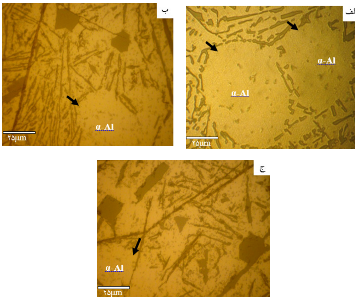
شکل ۹- مورفولوژی دانه‌های سیلسیم در حالت اعمال جریان الکتریکی. (الف) جریان الکتریکی مستقیم، (ب) جریان متناوب با شدت جریان ۲۷۵ آمپر و (ج) جریان متناوب با شدت جریان ۱۲۵ آمپر
