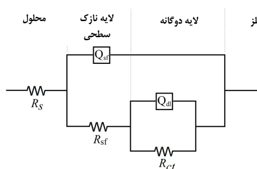
شکل ۸- مدار معادل الکتریکی منحنی امپدانس نمونه‌های آلومینیومی در محلول ۳/۵٪ کلرید سدیم.
