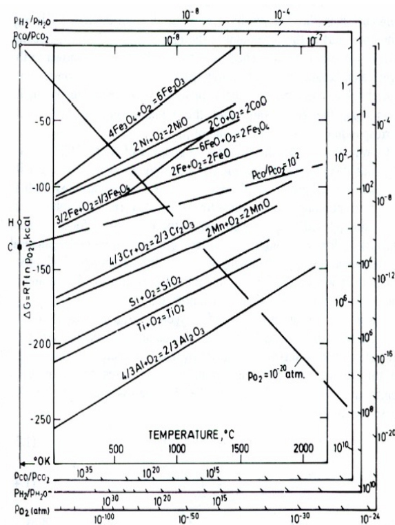
شکل ۳- دیاگرام الینگهام [۲۱].
