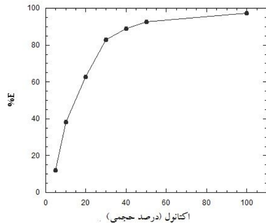
شکل ۱- تاثیر نسبت حجمی اکتانول/کروزن بر درصد استخراج
