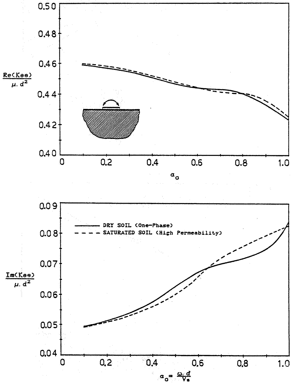
شکل ۱۲ - تأثیر نفوذ پذیری بر سختی دینامیکی افقی پی صلب
