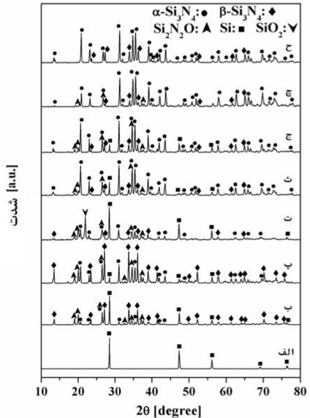
شکل ۱- الگوهای پرتو ایکس پودرهای الف) ماده اولیه سیلیسیم، ب) SN1، پ) SN2، ت) SN3، ج) SN4، ج) SN5، ح) SN6 و ح) SN7
