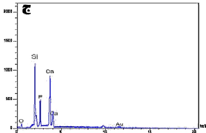
شکل ۲- تصاویر میکروسکوپی الکترونی روبشی از الیاف شیشه زیست فعال پس از الکتروریسی: الف) پیش از عملیات حرارتی با میانگین قطر ۱۳۹ نانومتر، ب) پس از عملیات حرارتی با میانگین قطر الیاف ۸۹ نانومتر و ج) تحلیل عنصری الیاف پس از عملیات حرارتی
