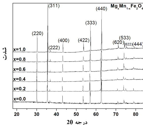
شکل ۳- الگوی پراش پرتو ایکس فریت Mg_xMn_{1-x}Fe_2O_4 در دمای تفجوشی ۱۲۵۰ درجه سانتی‌گراد
