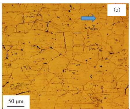
شکل ۱- ریزساختار Hastelloy X تحت عملیات حرارتی آیل در دمای ۱۱۷۵ درجه سانتی‌گراد: الف) فاقد منیزیم، ب) حاوی ۱۷ ppm، ج) حاوی ۳۳ ppm و د) حاوی ۴۷ ppm منیزیم
