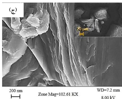
شکل ۲- تصاویر میکروسکوپی الکترونی روبشی نمونه‌های: الف) S_m ، ب) S_{am} و ج) S_{aa}
