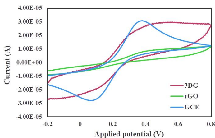
شکل ۱۰- منحنی آزمون ولتاژمتری چرخه‌ای الکتروود کربن شیشه‌ای، اکسید گرافن احیا شده و گرافن سه بعدی با نرخ اسکن ۱۰۰ میلی‌ولت بر ثانیه (رنگی در نسخه الکترونیکی)
