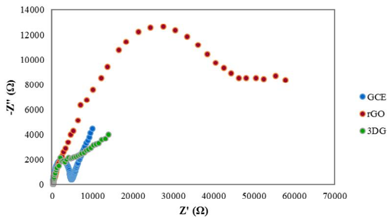
شکل ۸- نمودار امپدانس الکتروشیمیایی الکتروکود کربن شیشه‌ای، اکسید گرافن احیا شده و گرافن سه بعدی
