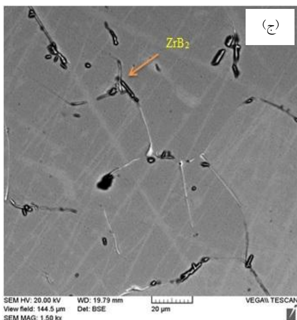
شکل ۳- تصاویر میکروسکوپی الکترونی روبشی آلیاژهای: الف) \text{Fe}_3\text{Al}-0.5\text{B} ، ب) \text{Fe}_3\text{Al}-0.5\text{Zr} و پ) \text{Fe}_3\text{Al}-0.5\text{Zr}-0.5\text{B}
