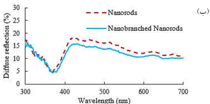
شکل ۷- طیف‌های: الف) بازتاب و ب) عبور پخش‌ی پوشش‌های متشکل از نانومیل‌ها و نانومیل‌های نانوبرگ‌دار شده دی‌اکسید تیتانیم
