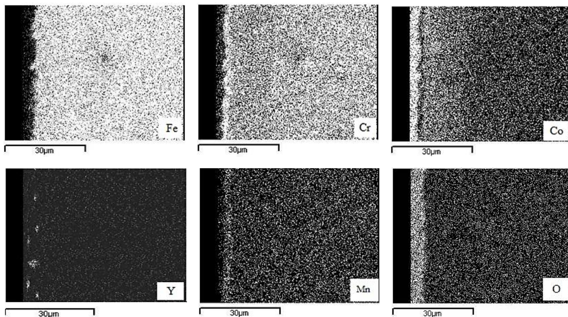
شکل ۱۰- آنالیز نقشه عناصر: الف) کبالت، ب) کروم، ج) آهن، د) اکسیژن، ه) منگنز و و) ایتريم از سطح مقطع فولاد Crofer22 APU پوشش داده شده با Co/Y_2O_3 بعد از ۵۰۰ ساعت اکسیداسیون همدمای در هوا در دمای ۸۰۰ درجه سانتی گراد
