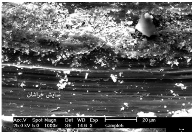
شکل ۵- تصاویر میکروسکوپی الکترونی روبشی از سطح سایش پین تحت بار ۳۰ نیوتن و مسافت ۱۰۰۰ متر برای:
