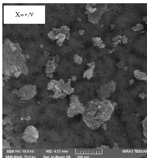
شکل ۳- تصاویر میکروسکوپی الکترونی روبشی نمونه‌های فریت کبالت آلاینش یافته با کروم به‌ازای درصدهای مختلف آلاینش
