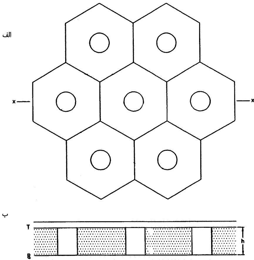
شکل ۲- مدل جریان پوسته‌ای الف: نمای بالا ب: سطح مقطع x-x
