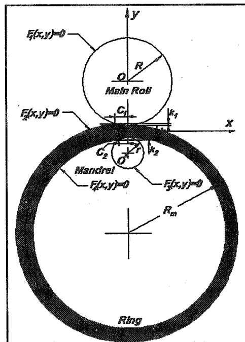
شکل ۴- معرفی ظوابط هندسه غلتکهای کار و حلقه
