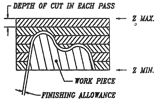
شکل ۱۳ - بعضی از پارامترهای تراش
