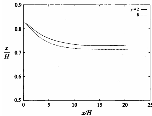
شکل ۱۷- اثر نسبت چسبندگی روی موقعیت تعادل برای یک قطره سه بعدی با We=0.5 و \alpha=\gamma=8 و Re=10 .
