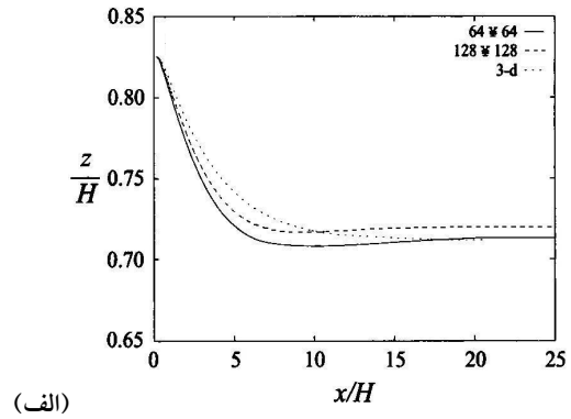
شکل ۱۶- مقایسه بین تشابه سازی دو بعدی و سه بعدی یک قطره در We=0.5 ، \alpha=\gamma=8 و Re=10 .
