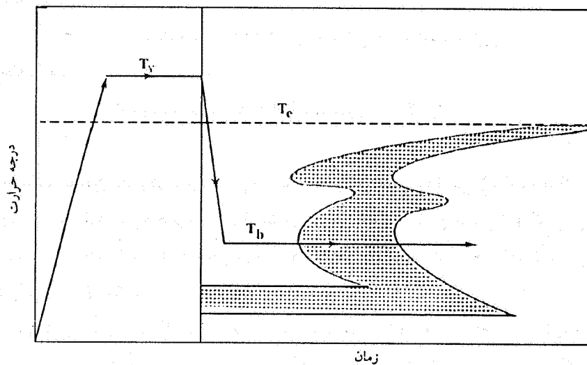
شکل ۱- نمودار عملیات حرارتی آستمپر کردن مخصوص چدنهای نشکن
