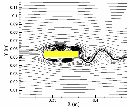
ج - c/t = 8
