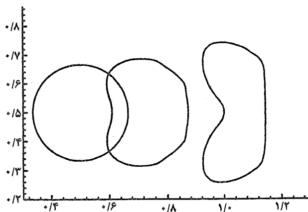
شکل ۱۲- تغییر شکل قطره در Re_l=200 و Re_g=10 در زمانهای t=0, 0.24, 0.6 و We=4
