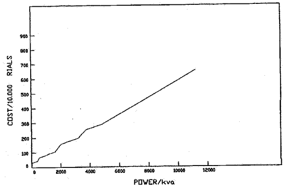
شکل ۳- هزینه پستهای فشار ضعیف برحسب قدرت آنها
