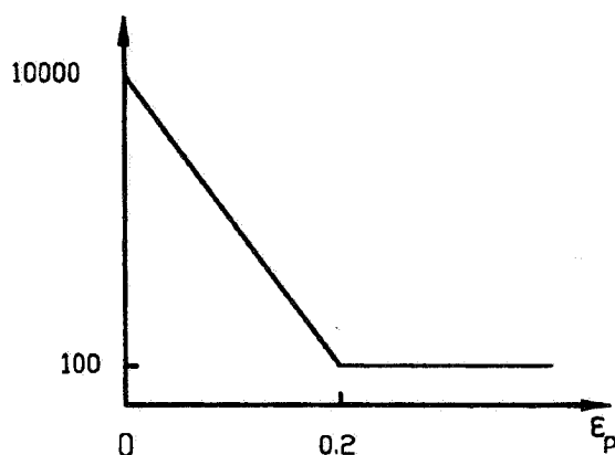
شکل ۴- تغییرات چسبندگی با \epsilon_p در مثال (۱)
