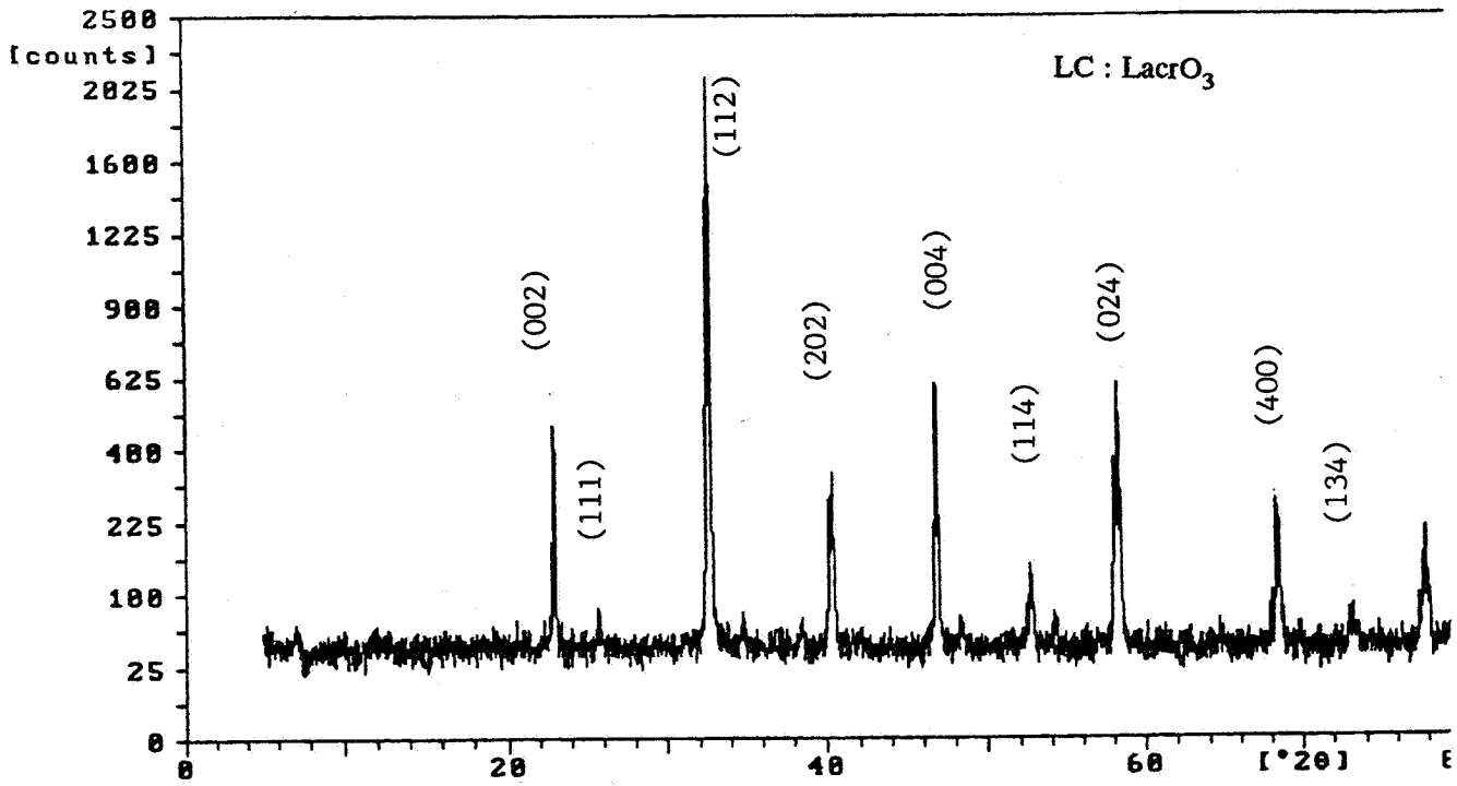
شکل ۶- الگوی پراش پرتو X ترکیب لاتانیم کرومیت کلوغه شده در دمای 1600^\circ\text{C}
