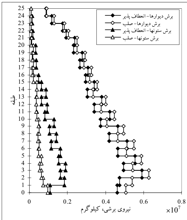
شکل ۱۲- مقایسه نیروی برشی دیوارها، ستونها و طبقه در تحلیل سازه با فرض دیافراگم‌های صلب و انعطاف‌پذیر، نمونه ۴
