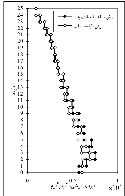
شکل ۱۲- مقایسه نیروی برشی دیوارها، ستونها و طبقه در تحلیل سازه با فرض دیافراگم‌های صلب و انعطاف‌پذیر، نمونه ۴
