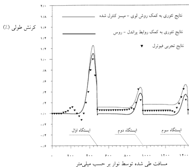
شکل ۸- نتایج تجربی فیوترل برای کرنش سنج شماره ۱ و نتایج تحلیلی برنامه تاجداری، برای کرنش طولی لبه [۱۰]
