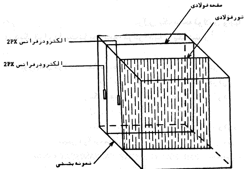
شکل ۱۵- موقعیت محل الکترودها ، تور و صفحه فولادی در بتن
