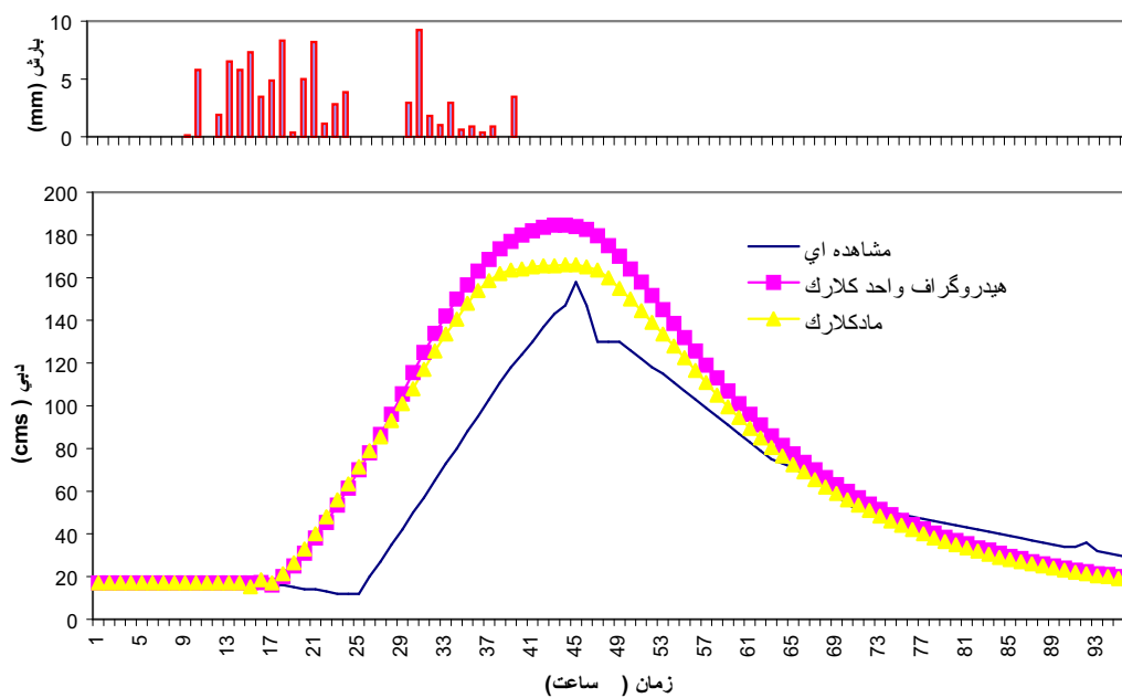
شکل ۴- مقایسه نتایج روش توزیعی - مفهومی ماد کلارک و روش هیدروگراف واحد کلارک در ایستگاه خرس آباد (سیلاب مورخ ۱ آذر ۷۳)
